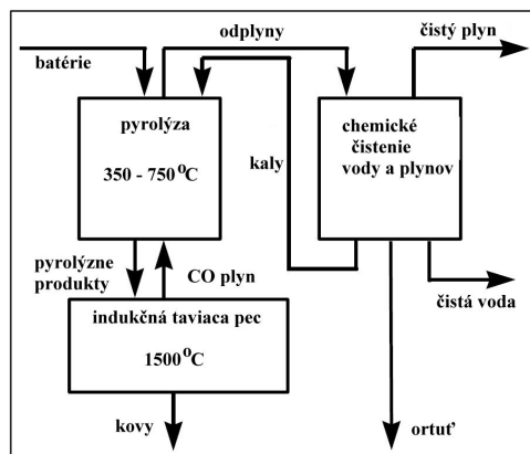
Obr.1 Bloková schéma recyklačného postupu Batrec
