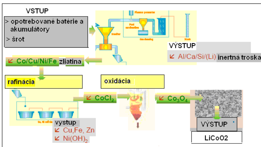
Obr.4 Bloková schéma recyklácie v procese Umicore
