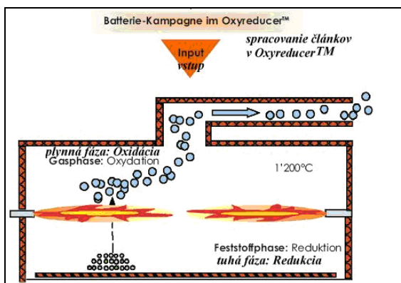
Obr.3 Proces Oxyreducer™ spoločnosti Citron
